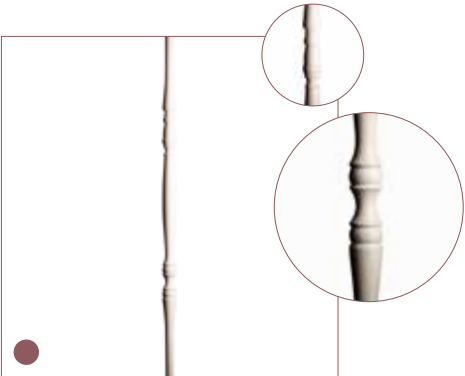
H-02 afwerking: voorgeschilderd, wit lengte: 970 mm doorsnede: Ø 22 mm gewicht: 0,35 kg afmeting sierwerk: 38 x 515 mm (bxh)
