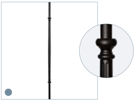
MR-02 HOL afwerking: gepoedercoat, mat zwart lengte: 970 mm doorsnede: Ø 16 mm gewicht: 0,68 kg afmeting sierwerk: 28 x 27 mm (bxh)
