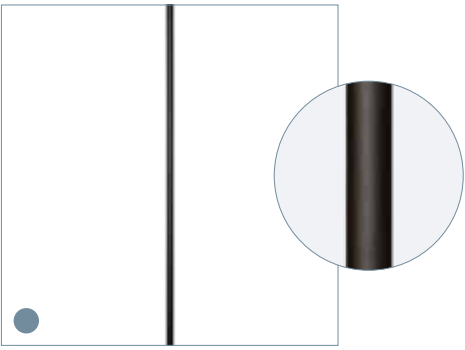
MR-07 MASSIEF afwerking: gepoedercoat, mat zwart lengte: 970 mm doorsnede: Ø 14 mm gewicht: 1,15 kg
