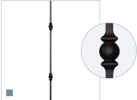
MV-06 HOL afwerking: gepoedercoat, mat zwart lengte: 970 mm doorsnede: 12,7 mm gewicht: 0,81 kg afmeting sierwerk: 25 x 51 mm (bxh)
