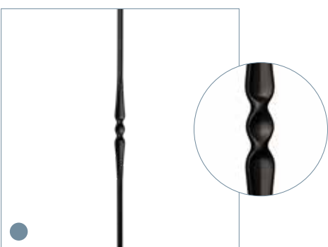
MR-08 MASSIEF afwerking: gepoedercoat, mat zwart lengte: 970 mm doorsnede: Ø 14 mm gewicht: 1,15 kg afmeting sierwerk: 26 x 295 mm (bxh)
