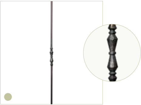
S-05 afwerking: warmgesmeed lengte: ±1.040 mm doorsnede: Ø 12 mm gewicht: 1,18 kg afmeting sierwerk: 26 x 130 mm (bxh)
