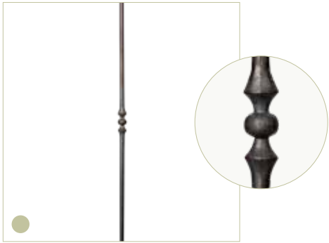
S-04 afwerking: warmgesmeed lengte: ±1.040 mm doorsnede: Ø 12 mm gewicht: 1,02 kg afmeting sierwerk: 24 x 65 mm (bxh)
