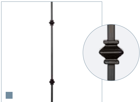
MV-08 HOL afwerking: gepoedercoat, mat zwart lengte: 970 mm doorsnede: 12,7 mm gewicht: 0,67 kg afmeting sierwerk: 40 x 40 mm (bxh)
