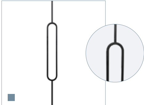
MV-15 HOL afwerking: gepoedercoat, mat zwart lengte: 970 mm doorsnede: 12,7 mm gewicht: 1,15 kg afmeting sierwerk: 95 x 525 mm (bxh)
