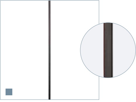
MV-01 HOL afwerking: gepoedercoat, mat zwart lengte: 970 mm doorsnede: 12,7 mm gewicht: 0,31 kg
