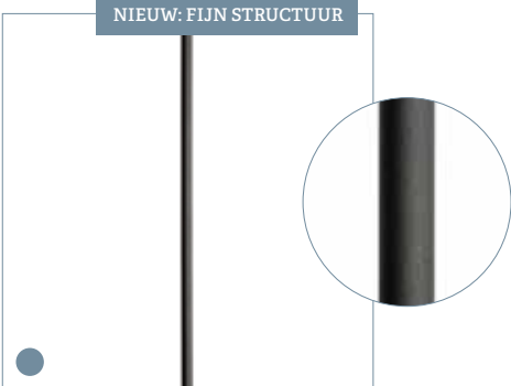
MR-07-S MASSIEF werking: gepoedercoat, fijn structuur mat zwart lengte: 970 mm doorsnede: Ø 14 mm gewicht: 1,15 kg
