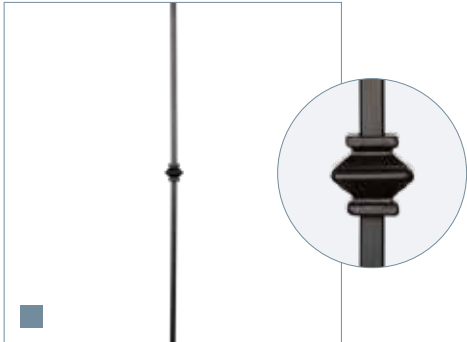
MV-07 HOL afwerking: gepoedercoat, mat zwart lengte: 970 mm doorsnede: 12,7 mm gewicht: 0,48 kg afmeting sierwerk: 40 x 40 mm (bxh)
