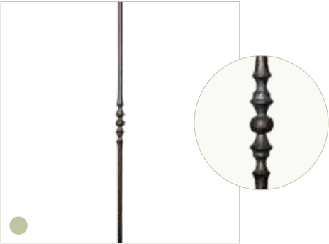
S-03 afwerking: warmgesmeed lengte: ±1.040 mm doorsnede: Ø 12 mm gewicht: 1,13 kg afmeting sierwerk: 25 x 112 mm (bxh)
