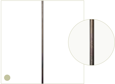
S-01 afwerking: warmgesmeed lengte: 1.000 mm doorsnede: Ø 12 mm gewicht: 0,89 kg
