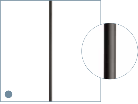
MR-11 MASSIEF afwerking: gepoedercoat, mat zwart lengte: 970 mm doorsnede: Ø 12 mm gewicht: 0,86 kg
