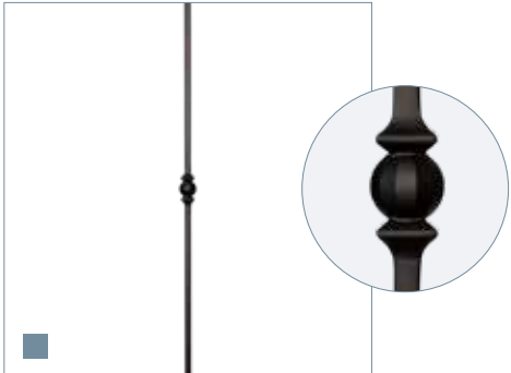
MV-05 HOL afwerking: gepoedercoat, mat zwart lengte: 970 mm doorsnede: 12,7 mm gewicht: 0,67 kg afmeting sierwerk: 25 x 51 mm (bxh)
