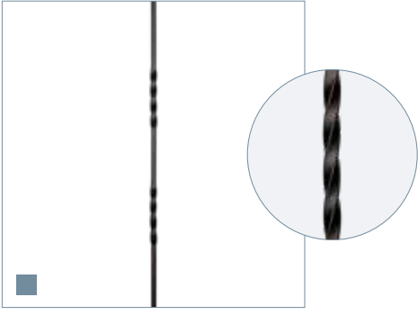
MV-04 HOL afwerking: gepoedercoat, mat zwart lengte: 970 mm doorsnede: 12,7 mm gewicht: 0,35 kg afmeting sierwerk: 12 x 152 mm (bxh)
