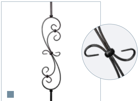
MV-13 HOL afwerking: gepoedercoat, mat zwart lengte: 970 mm doorsnede: 12,7 mm gewicht: 1,63 kg afmeting sierwerk: 147 x 599 mm (bxh)
