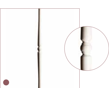
H-04 afwerking: voorgeschilderd, wit lengte: 970 mm doorsnede: Ø 22 mm gewicht: 0,31 kg afmeting sierwerk: 38 x 66 mm (bxh)
