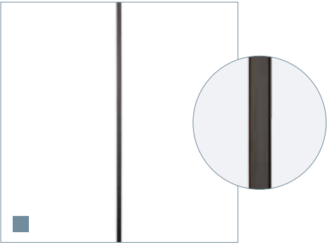
MV-02 HOL afwerking: gepoedercoat, mat zwart lengte: 1.125 mm doorsnede: 12,7 mm gewicht: 0,41 kg
